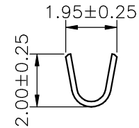
SEC:B-B
