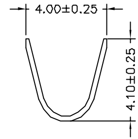
SEC:A-A
