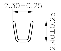
SEC:B-B
