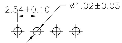
P.C.B LAYOUT
