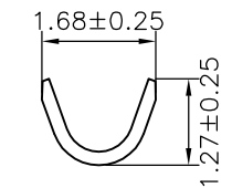
SEC:B-B
