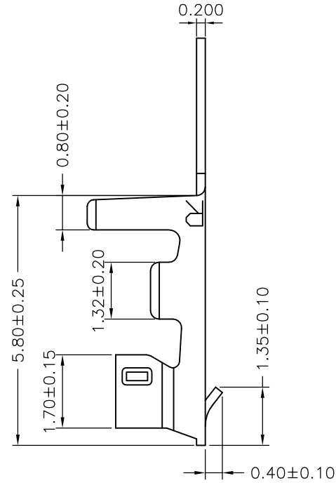
SEC:A-A
