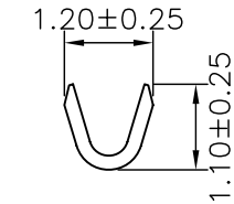
SEC:B-B
