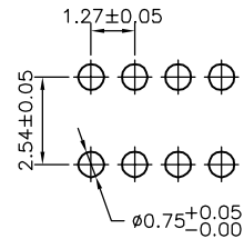
P.C.B LAYOUT
