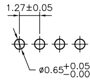
P.C.B. LAYOUT
